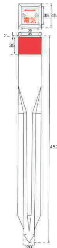
SUSポイント(R) 寸法図
